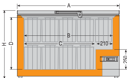
DIMENSIONI / SIZE / DIMENSIONS / MABE / MEDIDAS
